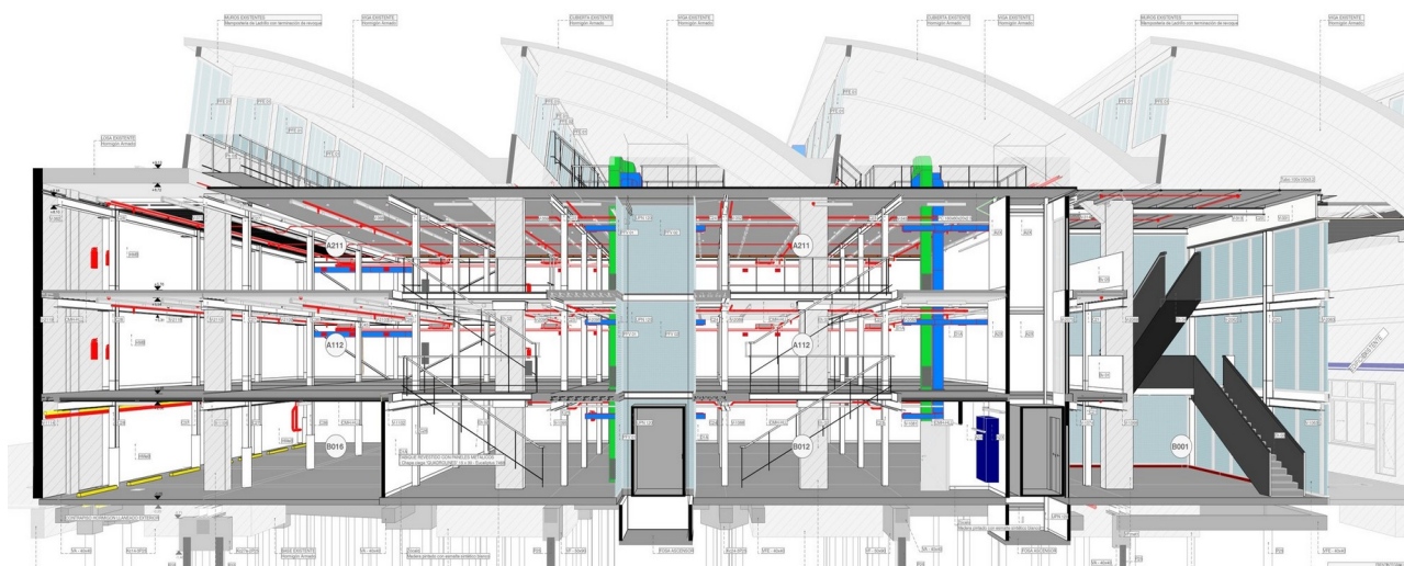
Nuevo Archivo del Poder Judicial de Santa Fe · corte del modelo federado · estructura, arquitectura e instalaciones sobre el edificio existente relevado · Archicad.
